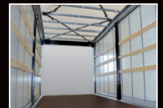
Curtainsider-Aufbau mit Schiebeplanen seitlich und Schiebendach zur Topbeladung
